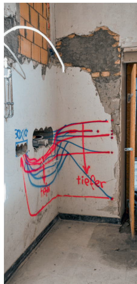
Im behutsam zu sanierenden historischen Gebäude ist auch das Anbringen der Kabelkanäle am richtigen Ort eine Arbeit, die Feingefühl erfordert. Das Ergebnis: eine spezielle Form der Graffiti-Kunst am Bau.
