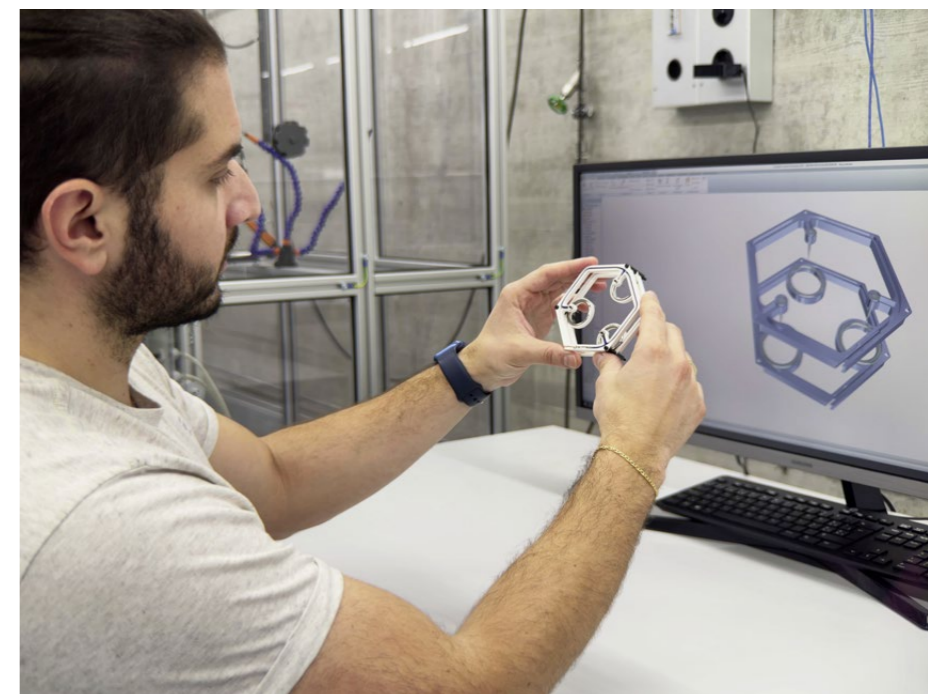
Der patentierte Luftstromverstärker des Empa-Spin-offs «Ionic Wind Technologies» beschleunigt Ionenwind viel stärker als bisher.
