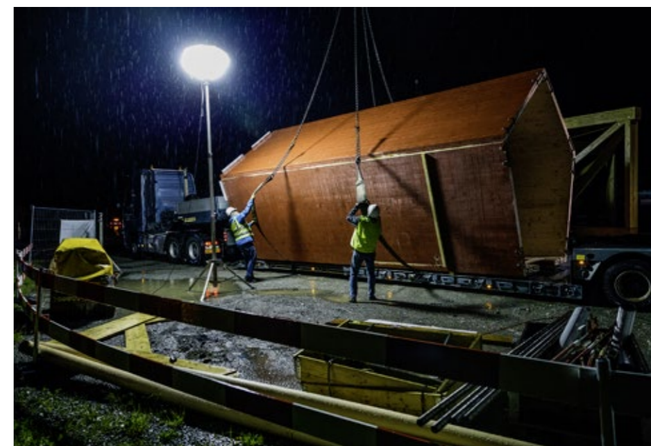
Die 40 Turmmodule wiegen bis zu 9,5 Tonnen und haben einen Durchmesser von 3,8 Metern.
